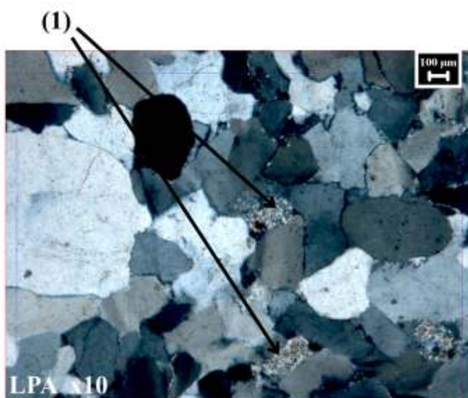
Photo 265 : Fantôme de grain de quartz (1) reconnaissable aux inclusions (petits points noirs) et à son contour d'origine marqué par une limite très fine et fugace (2). On observe au pourtour une frange de croissance epitaxique (par nourrissage secondaire du grain) relativement limpide (3) qui cimente le grain. Remarquer également, sur le pourtour de certains grains, une étroite zone a forte biréfringence (4) qui sera décrite avec la photo suivante.
