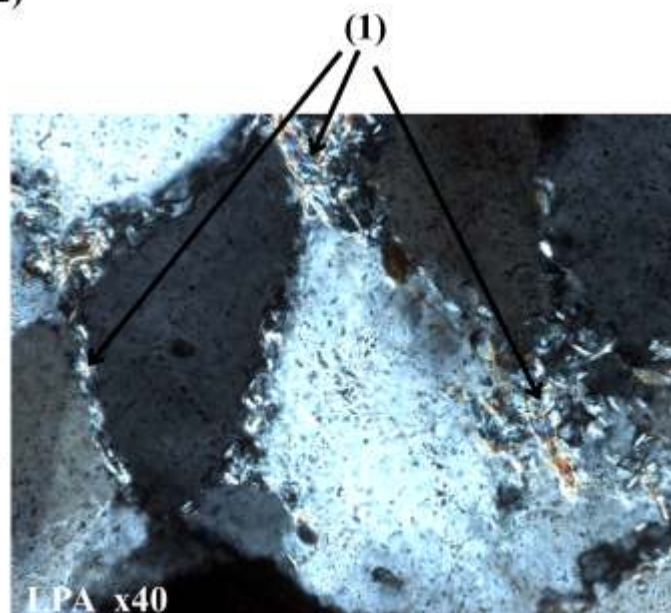
Photo 266 : Détail au très fort grossissement de la photo précédente (282) montrant la nature de l'étroite frange intergranulaire à forte biréfringence décrite ci-dessus. On constate qu'elle est constituée de fines paillettes ou lamelles enchevêtrées formant une sorte de joint entre les grains (1). Il est probable qu'il s'agisse d'argile néoformée selon un procédé de cimentation complexe par réaction intergranulaire.
