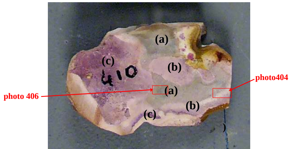
Photo 403 : Vue d'ensemble de la zone de prélèvement de la lame mince colorée au rouge d'alizarine. On distingue ce que l'on a observé sur le macro échantillon, savoir : une zone centrale (a) grise (non coloré par l'alizarine), un cortex subdivisé en une partie interne (b) rose pâle contenant une faible proportion de calcite et une partie périphérique (c) rose foncé ou violette entièrement carbonatée.
