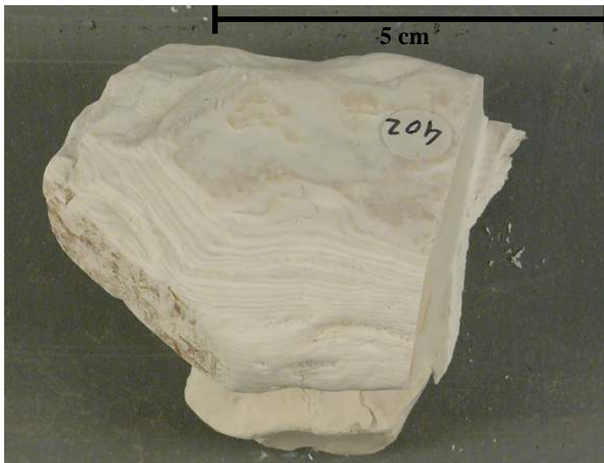
Photo 372 : Echantillon 402 de diatomite : roche claire très légère et friable, finement litée. Elle est formée de l'accumulation de tests (frustules) d'algues unicellulaires, les Diatomées . Ces frustules sont en silice, opale à l'origine.
