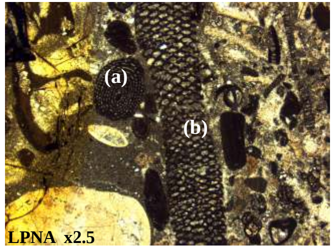
Photo 88 : Différentes coupes d'Alvéolines : (a) équatoriale, (b) axiale [voir schéma sur planche 75]. Remarquer ici aussi en (b), les loges centrales initiales à enroulement plus large.
