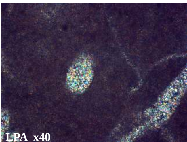
Photo 90 : Détail des photo précédentes au fort grossissement montrant la structure granuleuse des tests porcelanés des Alvéolines.
