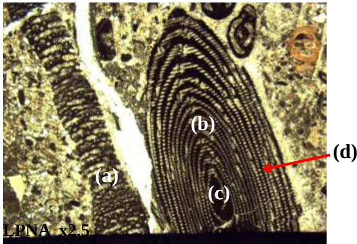
Photo 87 : Tests d'Alvéolines, (a) en section transverse ou axiale, (b) section circulaire ou équatoriale. On remarquera en (b) l'enroulement spirale des loges au début (c) large (loges initiales ou proloculus), puis serré par la suite. Les parois sont fines et gris sombre (d).
