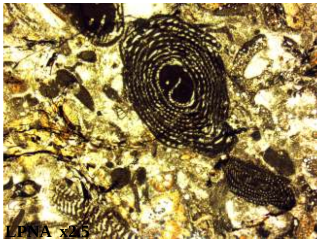
Photo 89 : Détail du début d'enroulement d'une Alvéoline à différents grossissements
