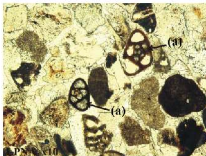
Photo 85 : Milioles (a) dans un micro faciès de roche calcaire
