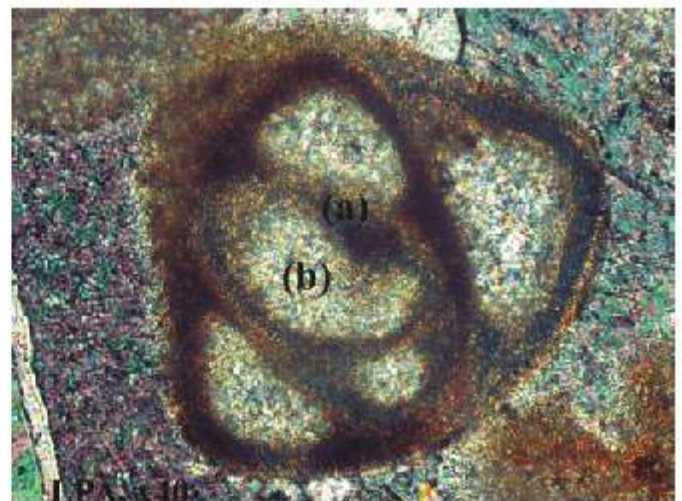
Photo 84 : Détail au fort grossissement de la photo précédente, montrant les parois (a) du test constituées d'une multitude de micro grains de calcite qui scintillent en LPA. Noter le remplissage postérieurement des loges (b) restées vide par un ciment de calcite limpide en mosaïque.
