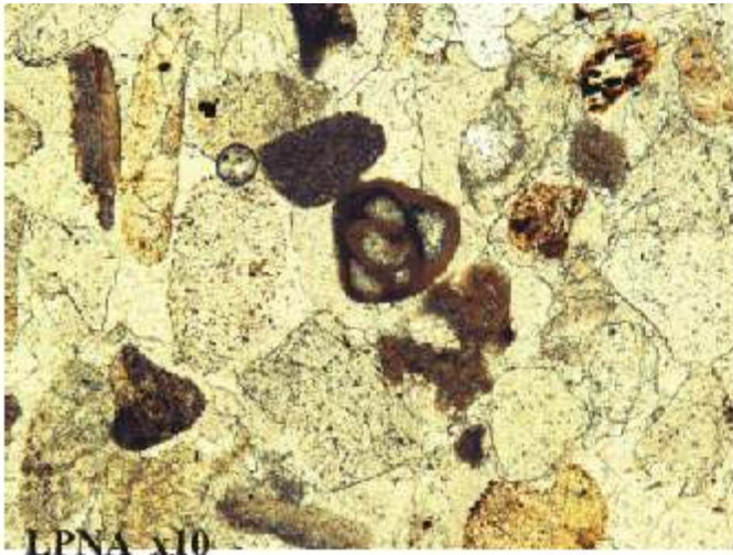
Photo 83 : Miliole , reconnaissable à la forme caractéristique (arquée) de ses loges et à la texture de son test porcelané, qui apparaît ici gris brunâtre à cause de la juxtaposition de micro grains de calcite mélangés à une composante organo ferrugineuse.
