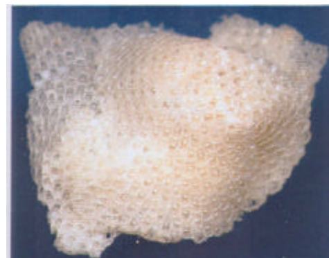
Squelette d'une colonie de bryozoaires actuels.
