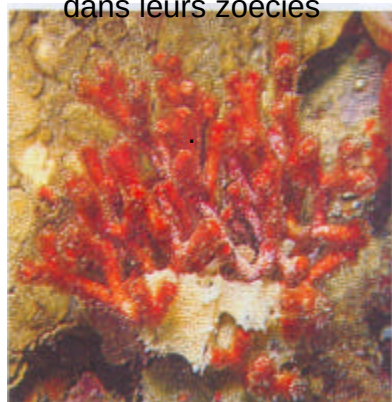
Détail de deux individus dans leurs zoécies
