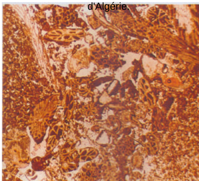
Faciès F4 - Packstone-Grainstone à bryozoaires et crinoïdes.
