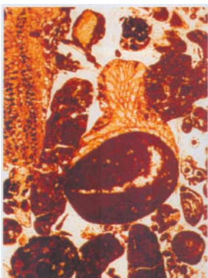
Bryozoaire fixé à un petit intraclaste arrondi.
