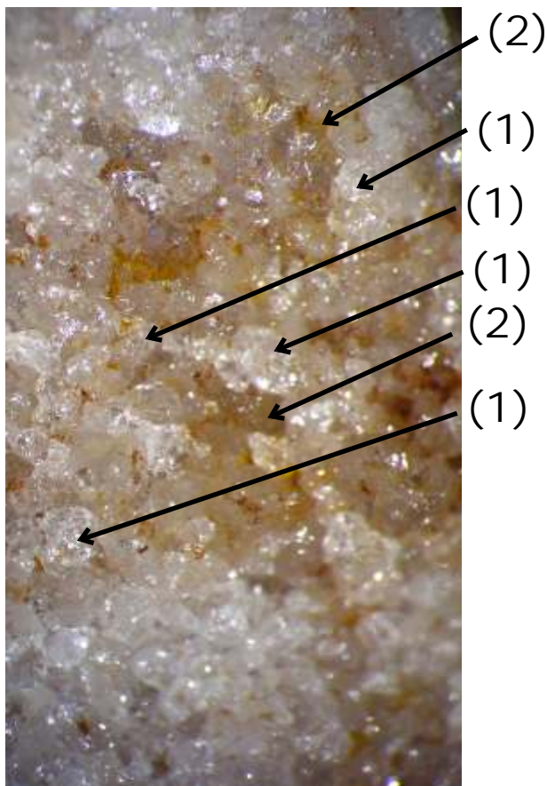
21_2 : Grès quartzite (photo x 1.6) détail montrant les grains de quartz en relief (<-- (1)) et la porosité (<-- 2)
