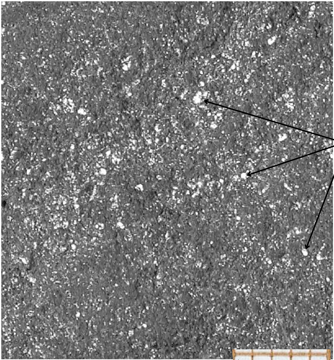
13_2 : Grès psammite ferrugineux (x 10)
