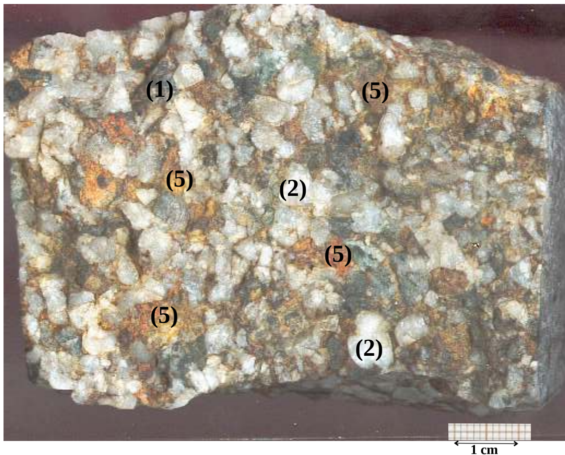
03_1 : Micro conglomérat grauwacke (x 1.7)
