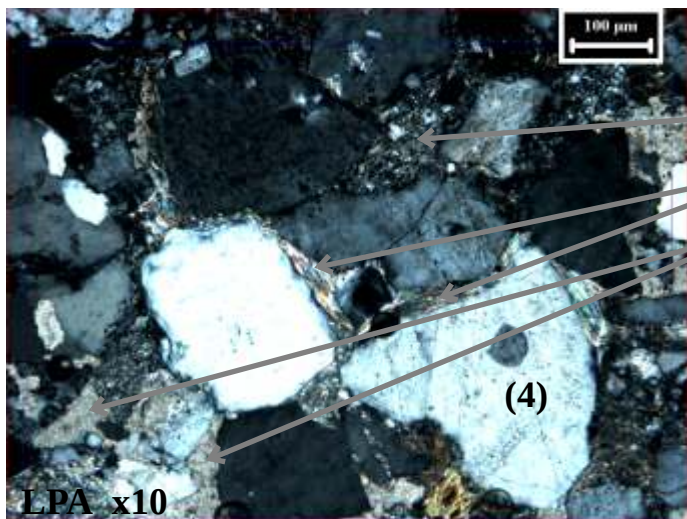
Photo 304 : Détail sur les différents types de phase de liaison rencontrés sur cette lame. (1) ciment de sparite, (2) argile fibreuse à forte biréfringence, (3) argile déstructurée grise mélangée à des fragments de minéraux. remarquer le quartz (4) avec une tourmaline en inclusion.
