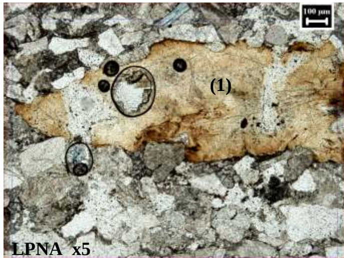
Photo 303 : Fragment de résine ou ambre de teinte brun jaune en LPNA (1) et isotrope en LPA(2).
